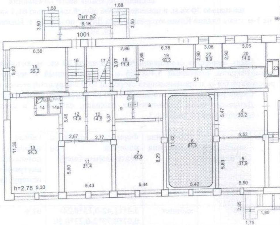
Рисунок 1 – схема расположения помещения №6 на поэтажном плане
